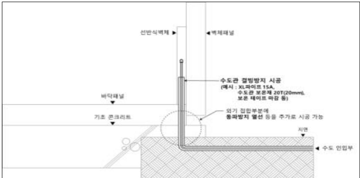
[수도관 결빙방지 시공 개략도]
