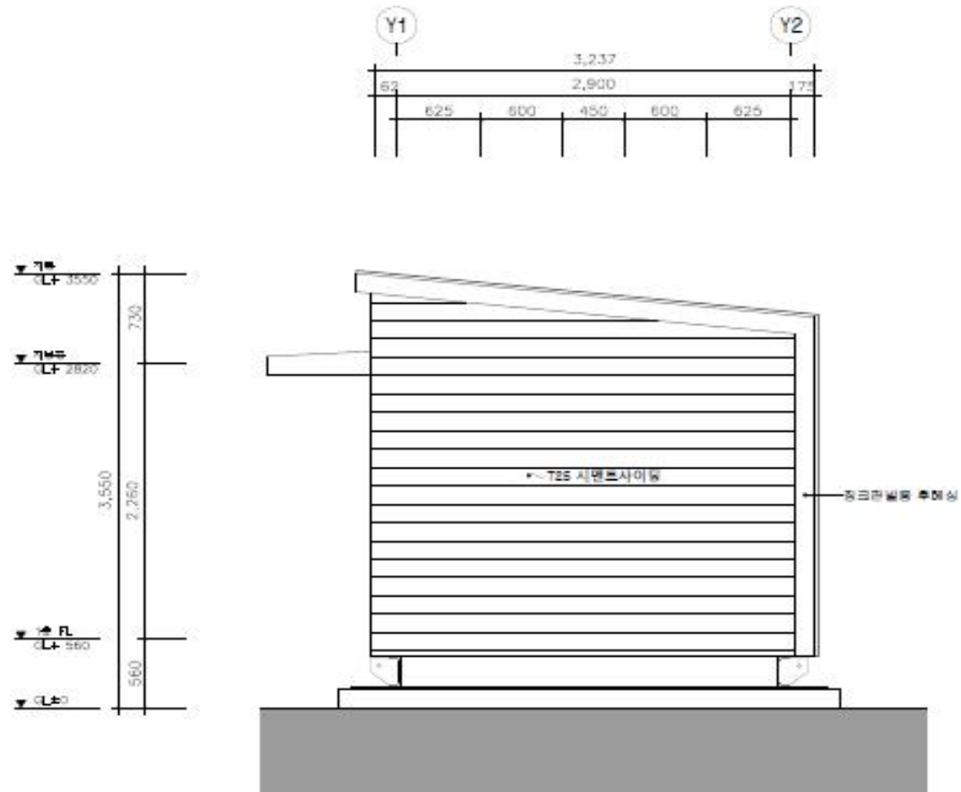
⑦ 좌측면도
